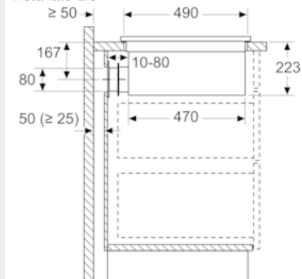
Dimensioni in mm Vista laterale
