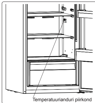
Temperatuurianduri piirkond
