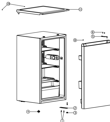
Frigorifero con pannello di copertura
