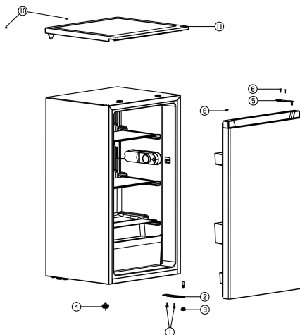
Koelkast met afdekpaneel
