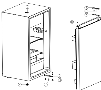
Koelkast zonder afdekpaneel
