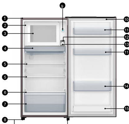
Geräteansicht
