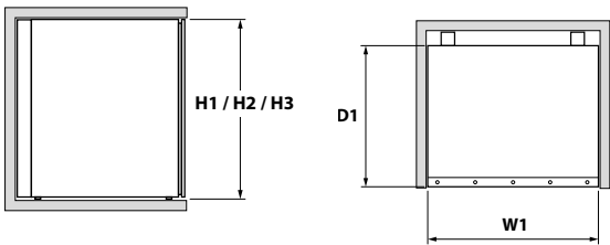
Dimensões totais
