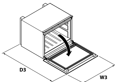
Totale benodigde afmetingen
