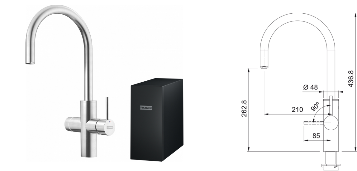
Miscelatore elettronico multifunzione MYTHOS WATER HUB SPARKLING
