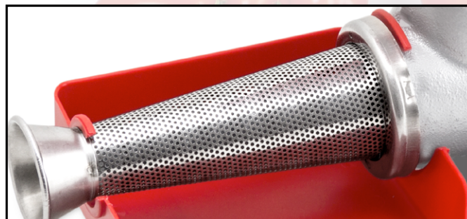
Cono filtro in acciaio inox 18/10 (AISI 304).
