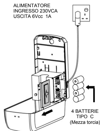
F Installazione batterie o utilizzo di alimentatore esterno
