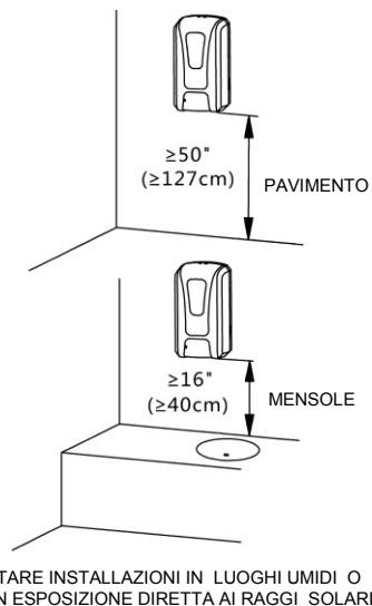
C Distanze di fissaggio consigliate
