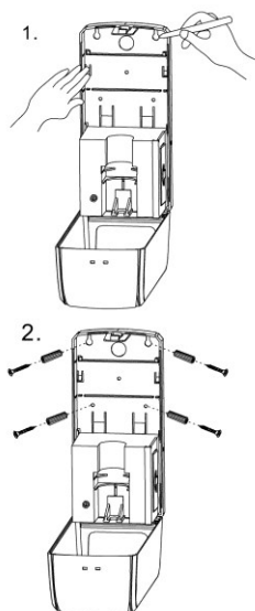
D Fissaggio a parete con viti e tasselli
