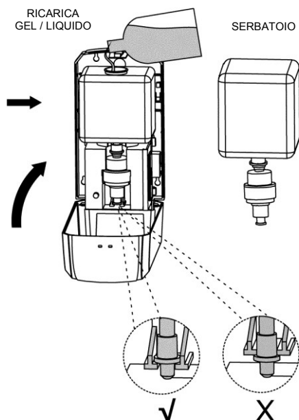
G Riempimento serbatoio
