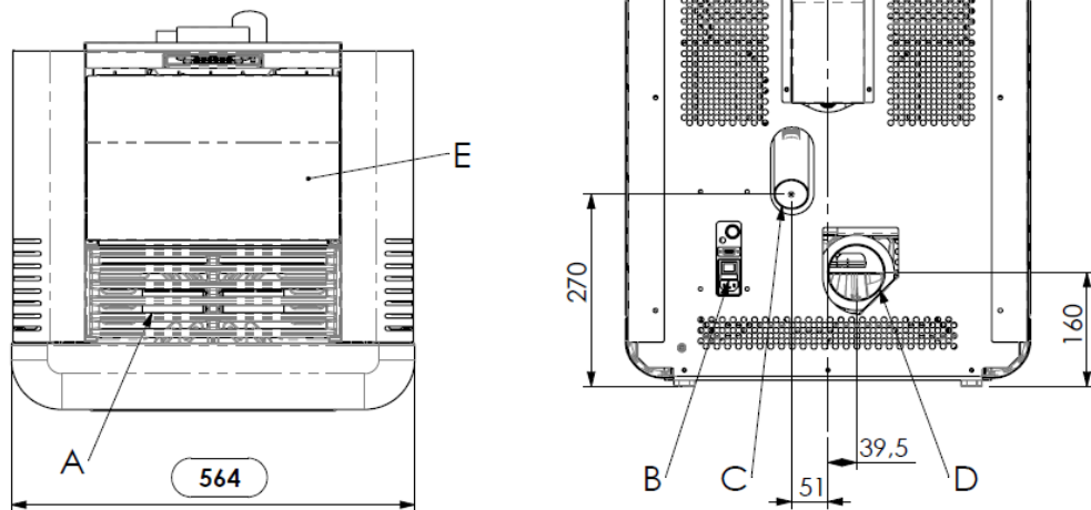
Abmessungen Pelletofen MEDEA LUX
