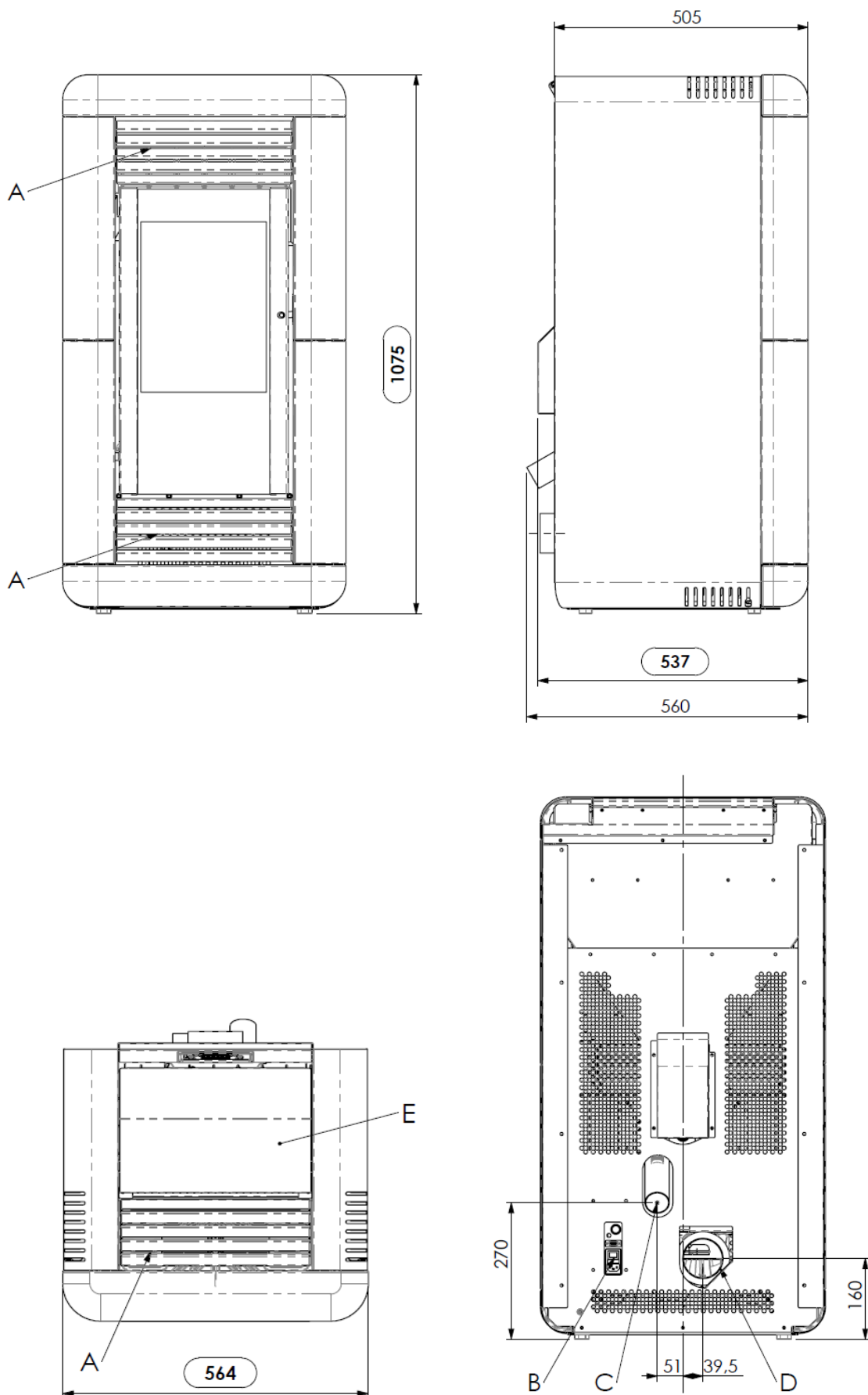
Ingombri stufa pellet Medea
