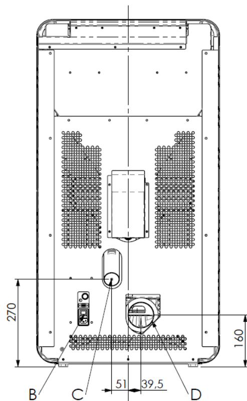
Abmessungen Pelletofen MEDEA
