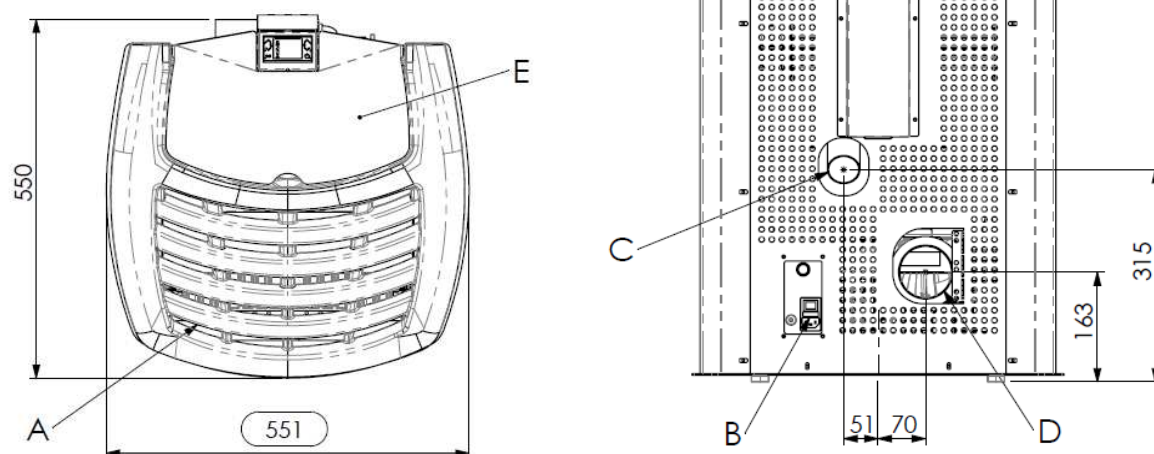
Ingombri stufa pellet DIAMOND
