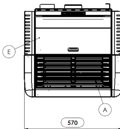
Medidas de la estufa de pellets CALLA canalizzabile
