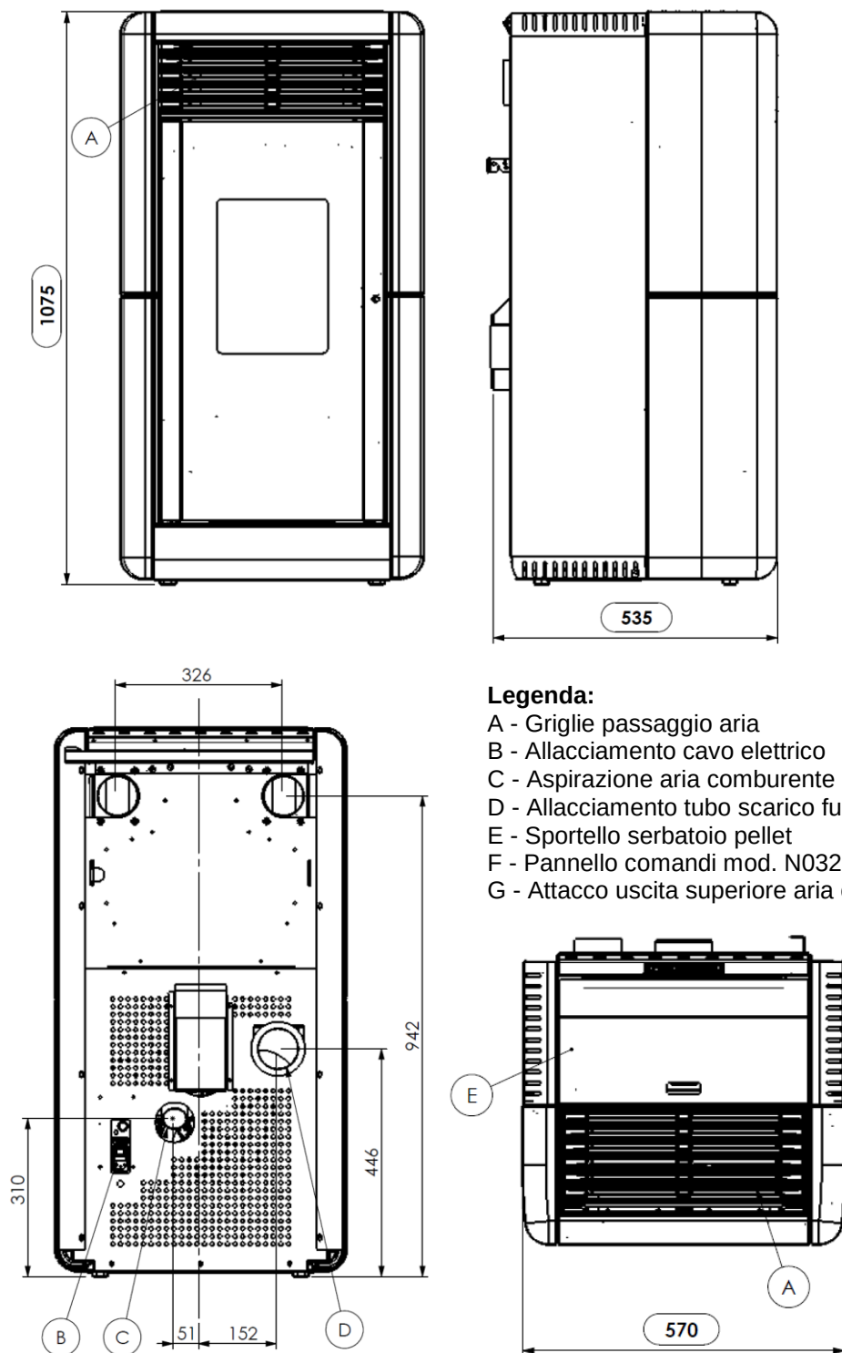
Ingombri stufa pellet CALLA canalizzabile
