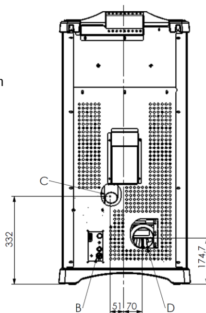
Ingombri stufa pellet ANTIGUA
