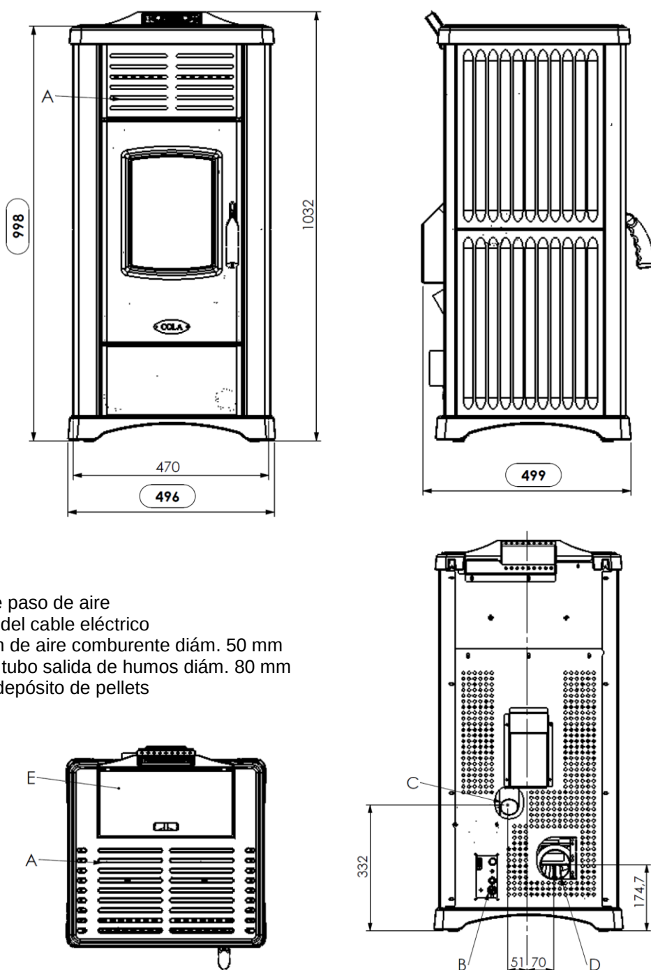
Medidas de la estufa de pellets ANTIGUA
