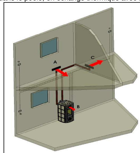
A – flux arrière air chaud canalisation gauche ; B – flux central air chaud ambient généré par le ventilateur central ; C – flux arrière air chaud canalisation droite ; a – thermostat extérieur local canalisation A ; b – sonde extérieure ambiance B implantation poêle ; c – thermostat extérieur local canalisation C ;
