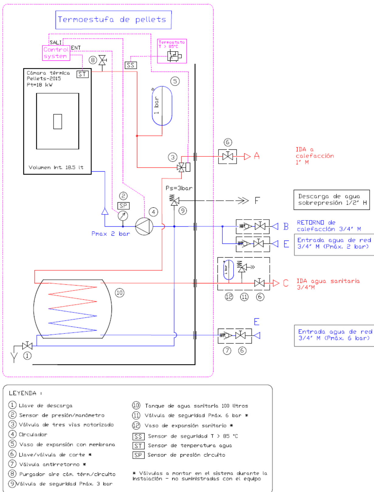
Esquema hidráulico de la termoestufa de pellets 18 kW_04-2015
