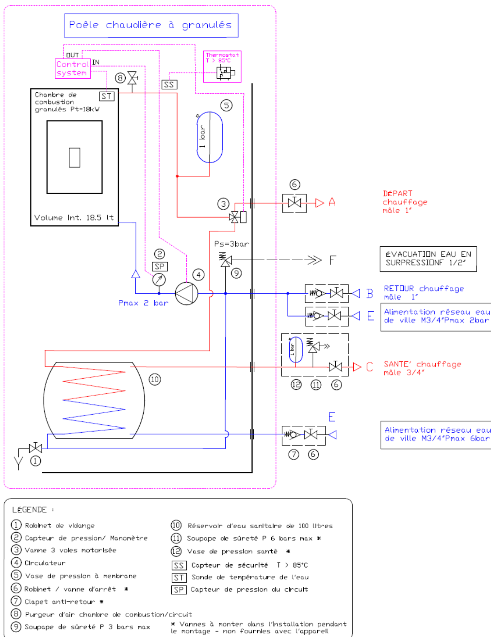
Schéma hydraulique du poêle chaudière à granulés 18 kW_04-2015
