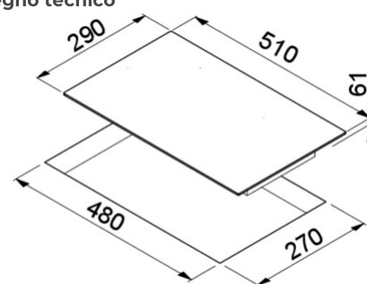
Disegno tecnico
