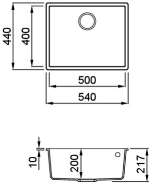
Disegno tecnico
