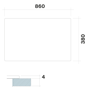
Installazione in appoggio
