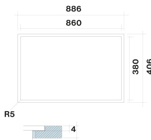
Installazione a filo
