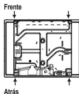
Posição do gancho para H=30mm
