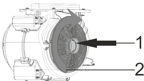
Fig. 10: FILTRO A CARBONI
