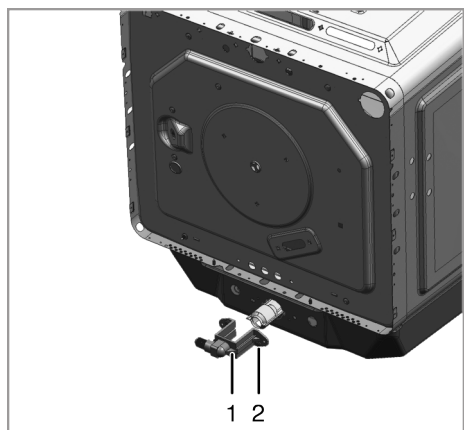
1 Supporto per iniettori 2 Vite
