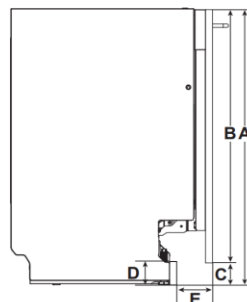
Immagine 1: Dimensione massima del pannello con cerniere fisse
