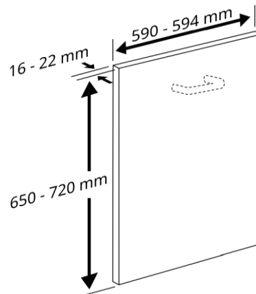
Immagine 1: Dimensione massima del pannello con cerniere fisse
