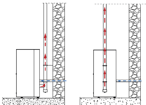
Installazione tipo "a" *
