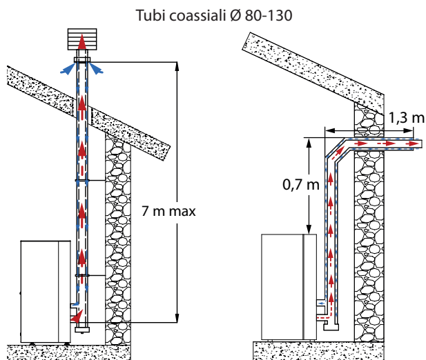
Installazione coassiale tipo "c" e "d" (dove previsto) *
