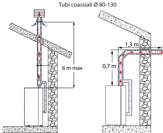
Installazione coassiale tipo "e" e "f" con accessorio (dove previsto) *
